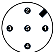
LED-Statusleuchte mit M12 Stecker (RGB)
