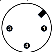
LED-Maschinenleuchte mit M12 Stecker (Weißlicht)
